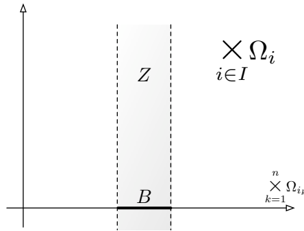
Abbildung 2: Zur Definition von Zylindermengen: Eine Zylindermenge ist stets durch Bedingungen an nur endlich vielen Komponenten ihrer Elemente definiert.
