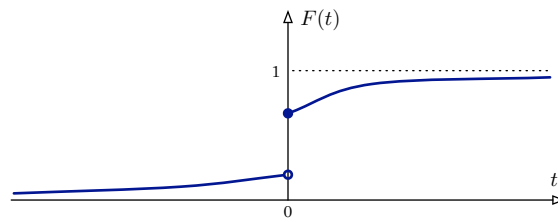
Abbildung 1: Zum Beispiel (2.2.2.1) einer Verteilungsfunktion.
